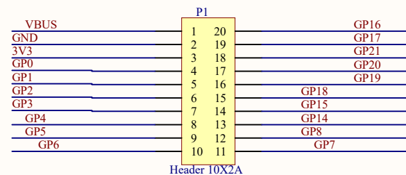
Header 10X2A
